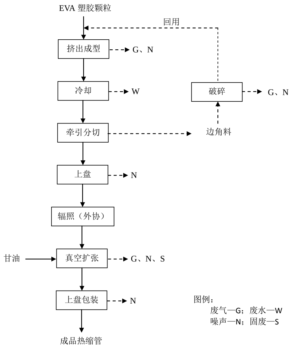
图3 本项目热缩管生产工艺流程及污染节点图
