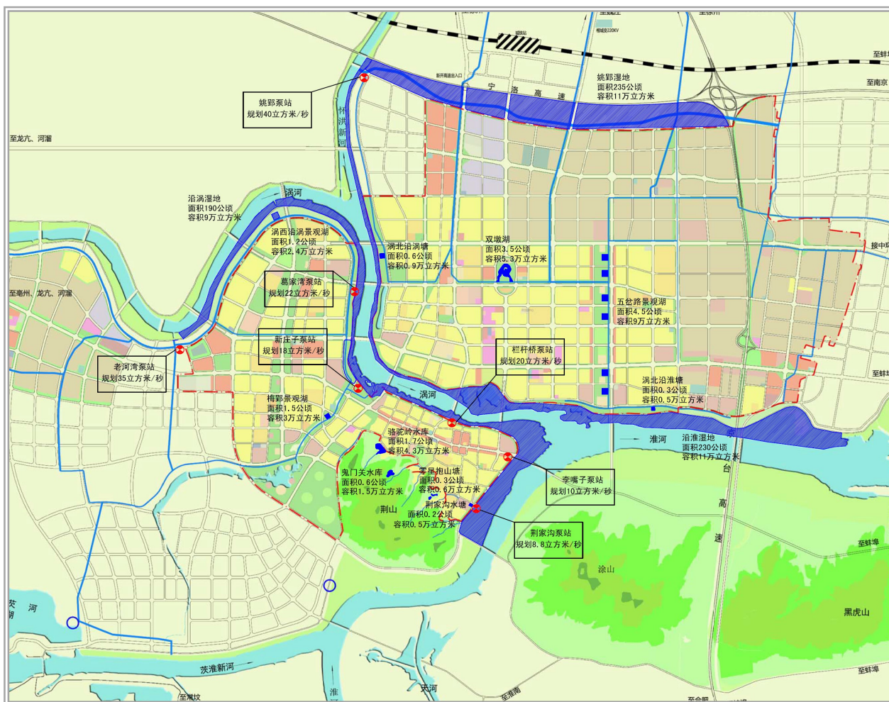
图 6-5 怀远县城区调蓄水体规划图
