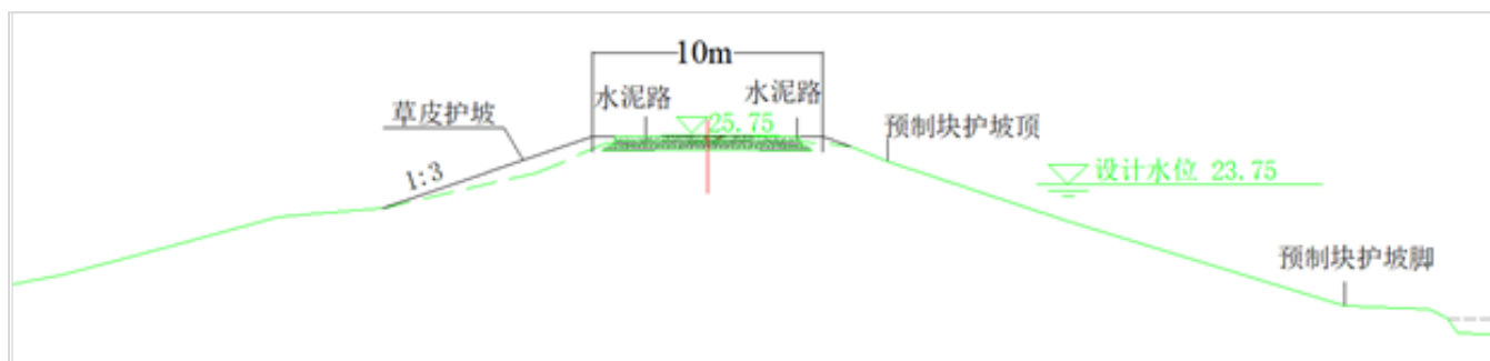
图 5-2 塌荆段堤防加固断面示意图
