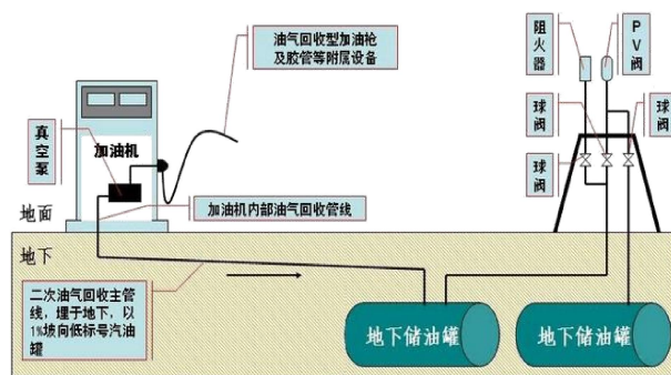
图 2-4 加油站汽油加油油气回收系统示意图
