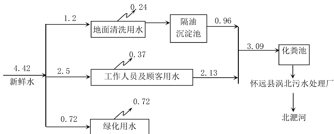
图 4-1 水平衡图 (m³/d)
