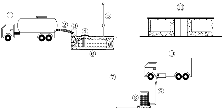
图 2-2 加油站工艺流程图
