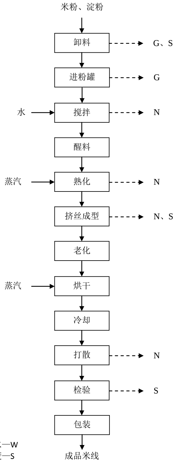
图 3 本项目米线工艺流程及污染节点图
